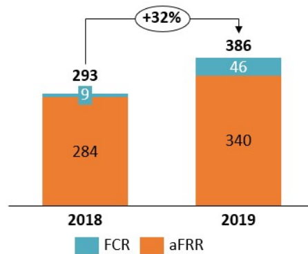
A szabályozó központ által értékesített villamos kapacitás 2018 és 2019 években (aFRR: GWh; FCR: GWh sym )
